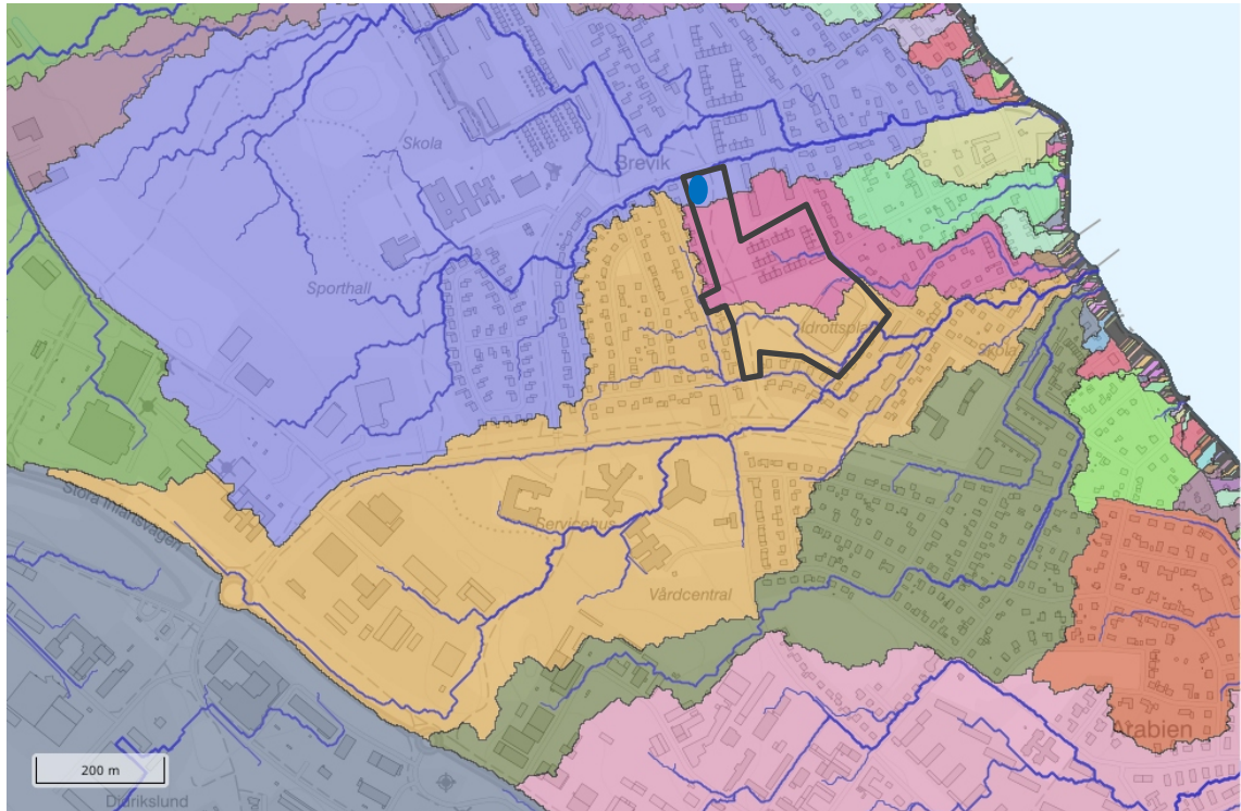
Figur 14. Översikt större avrinningsområden som berör planområdet markerat i svart. Födröjningsmagasinets ungefärliga placering markerad i blått (Dagvattenutredning, Tyréns).
