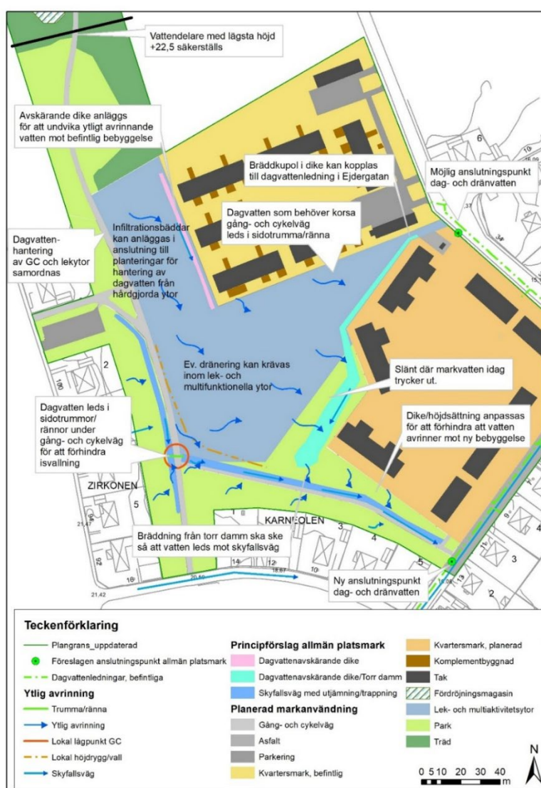
FIGUR 14: Förslag till principlösning för dagvatten- och skyfallshantering inom allmän platsmark (Tyréns, 2020).
