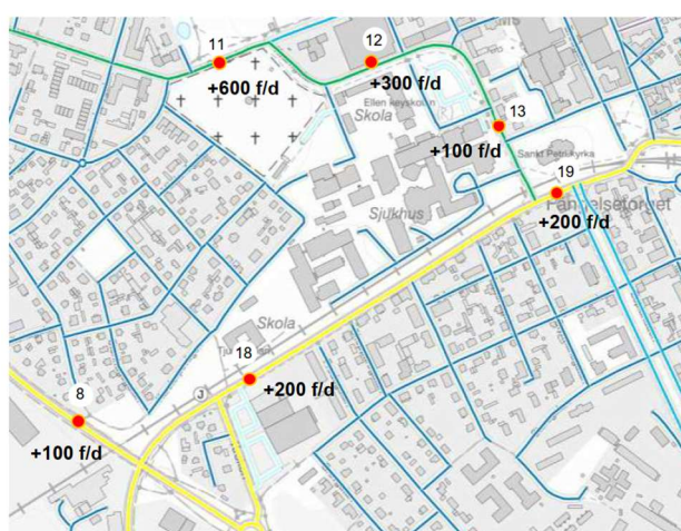
Figur 46 och 47 Förändring av förväntade trafikflöden omkring sjukhuset år 2040, utan respektive med ny södra infart
