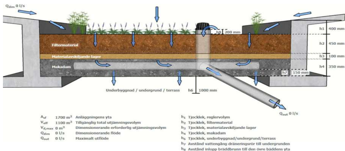
Figur 33: Principskiss på regnbädd.
