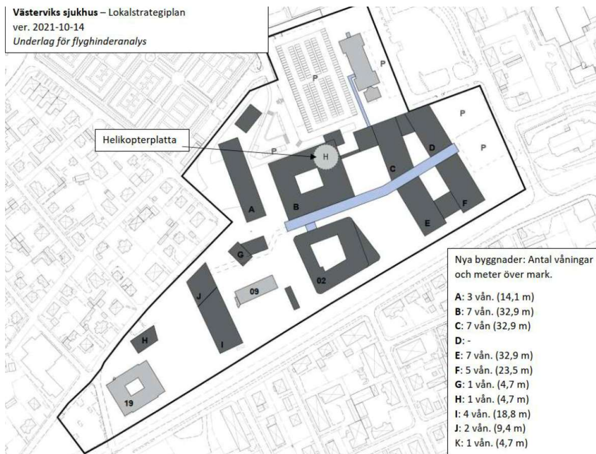
Figur 65: Höjd på planerade byggnader enligt LOST 2021. Planerad helikopterplatta på ny byggnad B.
