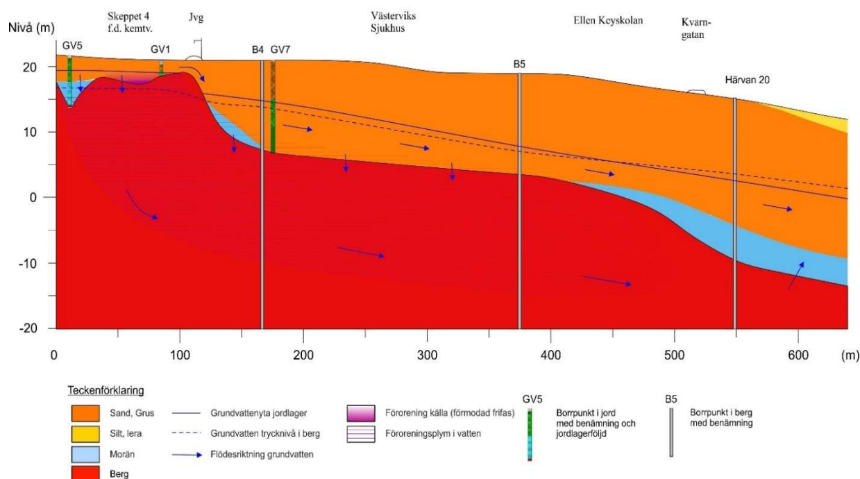
Figur 23. Konceptuell modell över hydrogeologiska förhållanden längs tvärsnitt B, från söder till norr (se Figur 21) med spridningsförhållanden för förorening från f.d. kemtvätt Skeppet 4. Referens: Rapport Structor juni 2024.
